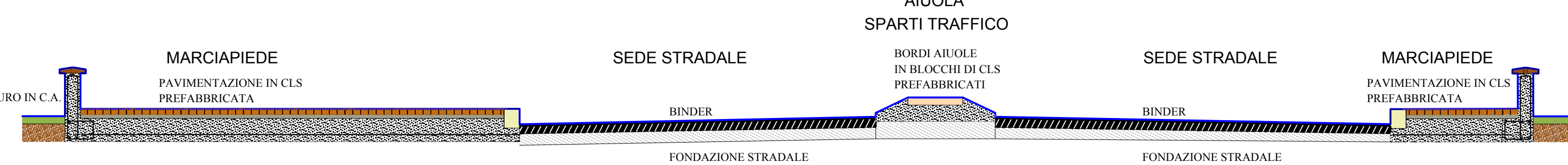
SEZIONE "B" ISOLE SPARTITRAFFICO rapp. 1: 50
