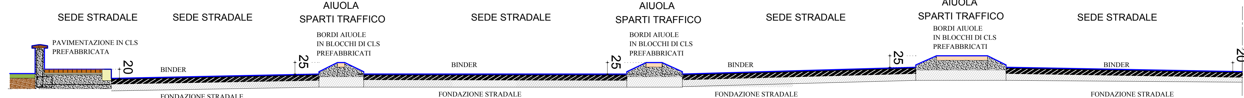
SEZIONE "C" ISOLE SPARTITRAFFICO rapp. 1: 50
