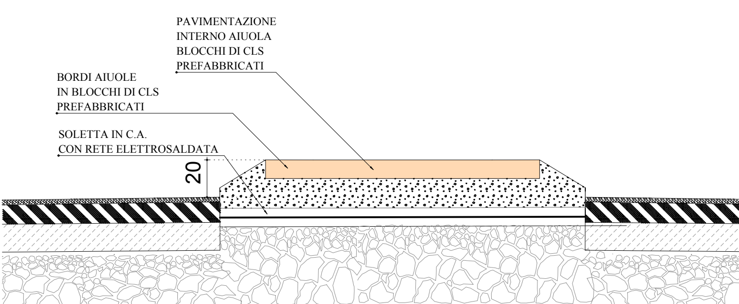
PARTICOLARE COSTRUTTIVO ISOLE SPARTITRAFFICO rapp. 1: 20
